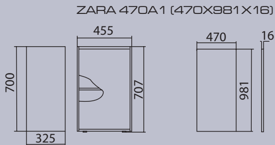
ZARA 320 (320X455X707)
